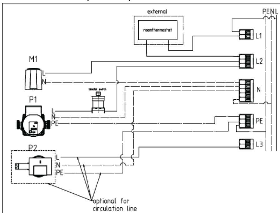
Collegamenti elettrici (esempio)
