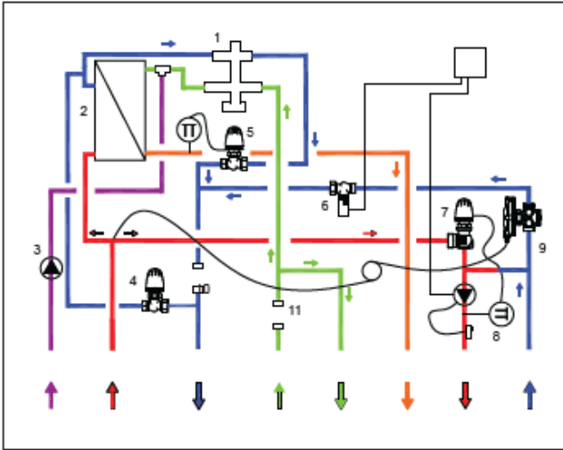
HIU Slovakia NT con ricircolo – Reg. Termostatica
