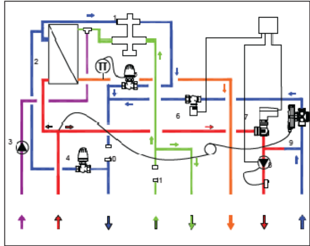
HIU Slovakia NT con ricircolo – Reg. Servomotore
