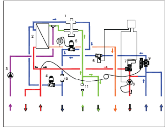
HIU Slovakia NT/HT con ricircolo – Reg. Servomotore
