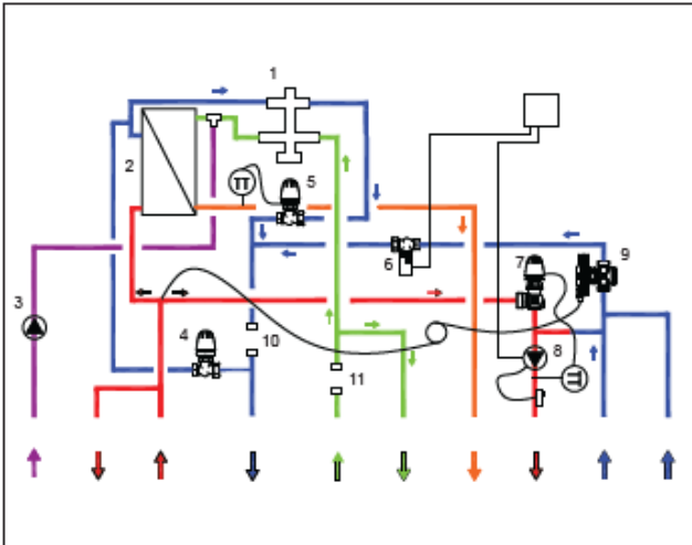
HIU Slovakia NT/HT con ricircolo – Reg. Termostatica
