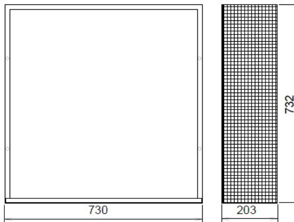
CASSERO IN LAMIERA ZINCATO COMPLETO DI RETE ESTERNA
